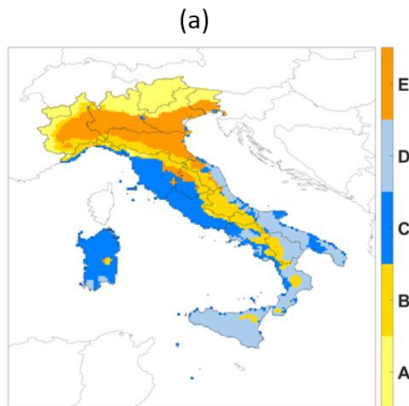
Figura 1.1-6: Scenario RCP8.5: (a) Mappa dei cluster individuati,
