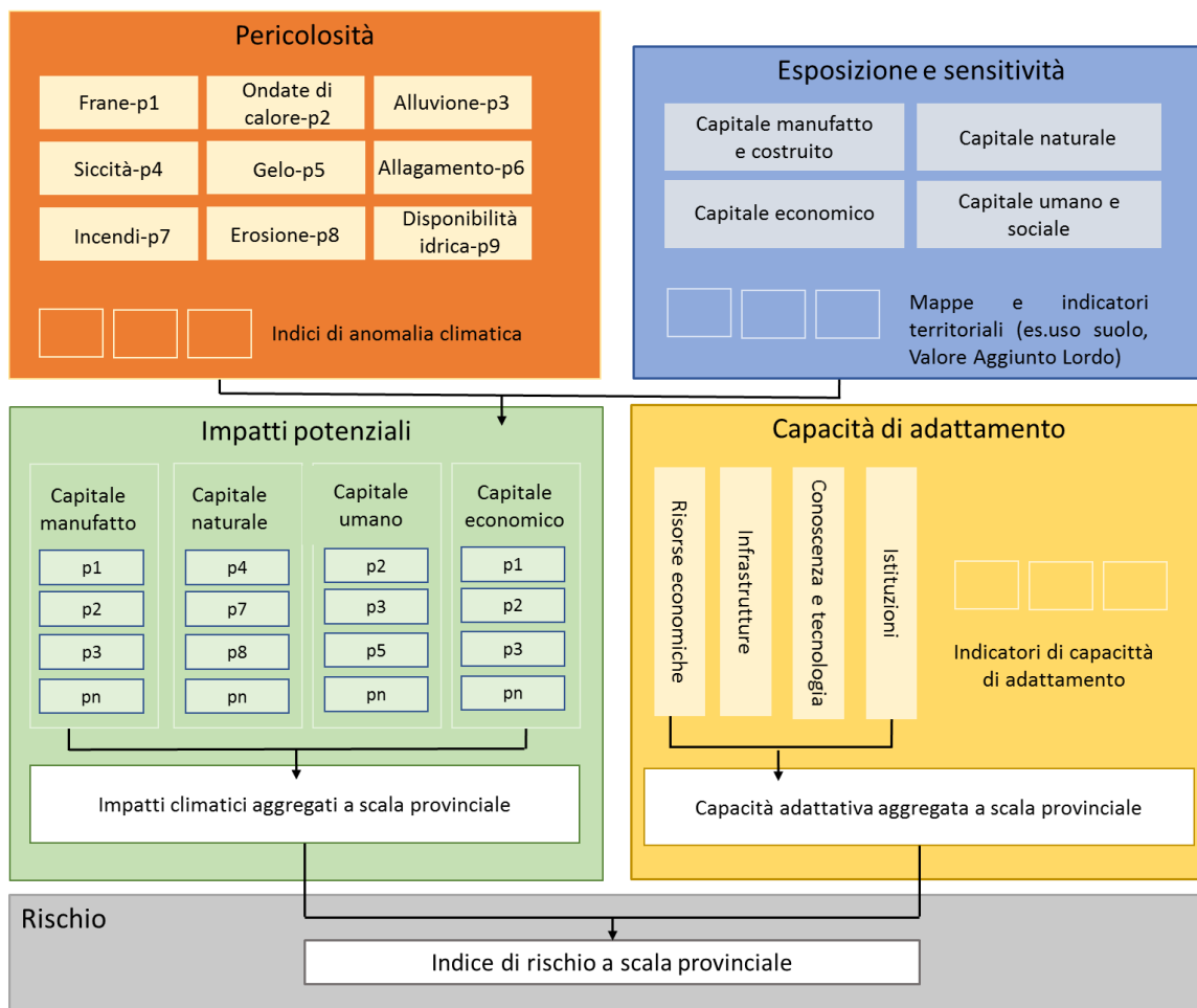
Figura 1.1-19: Schema dell'approccio metodologico applicato per il calcolo dell'indice di rischio.
