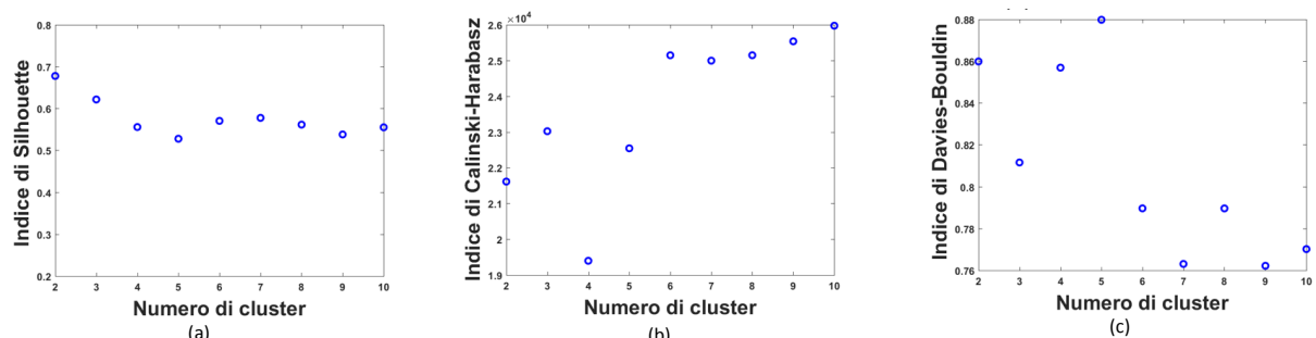
Figura 1.1-15: Metriche per l'identificazione del numero di cluster calcolate per il dataset MEDSEA RCP8.5 (box Mediterraneo centrale): (a) Indice di Silhouette, (b) Indice di Calinski-Harabasz, (c) Indice di Davies-Bouldin.
