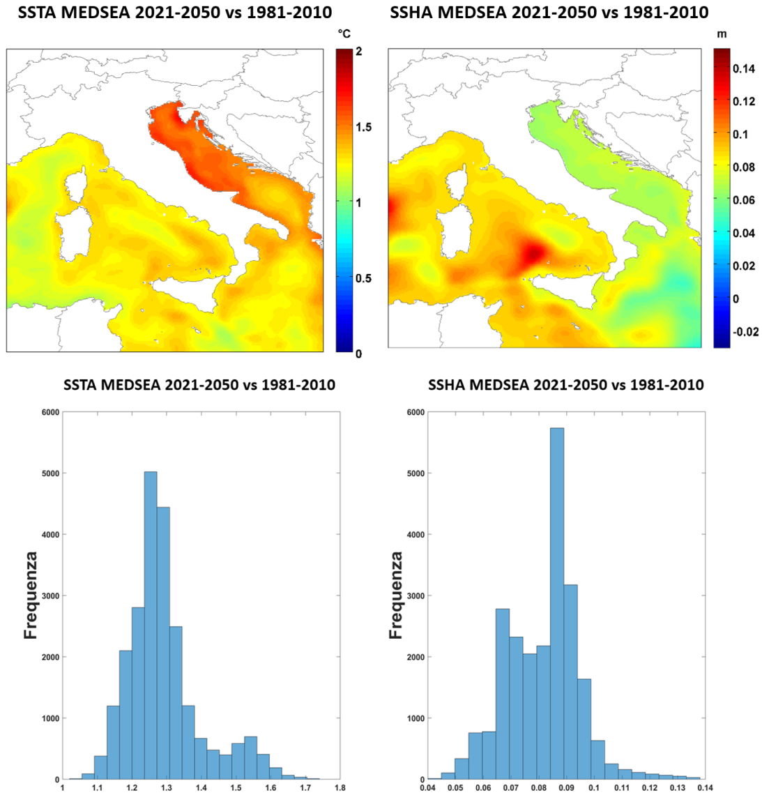
Figura 1.1-14: Climatologie degli indicatori SSTA e SSHA (pannelli superiori) e relative distribuzioni di frequenza (pannelli inferiori) sul Mediterraneo centrale ottenute dal dataset MEDSEA RCP8.5 per il periodo 2021-2050 vs 1981-2010).
