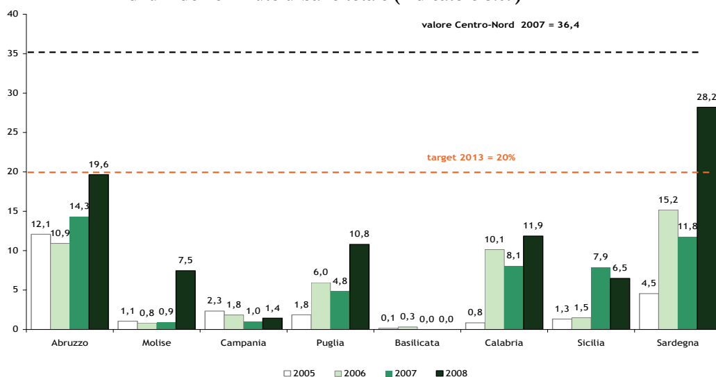
Figura III.11 Percentuale di frazione umida trattata in impianti di compostaggio sulla frazione di umido nel rifiuto urbano totale (indicatore S.09)
