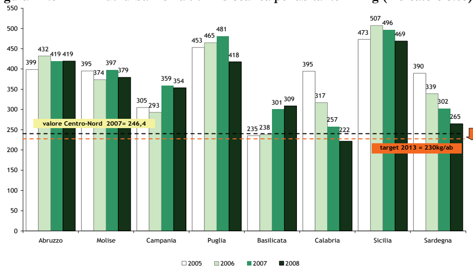
Figura III.8 Rifiuti urbani smaltiti in discarica per abitante - in kg (indicatore S.07)
